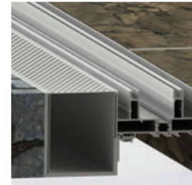
05 - Seuil Drainant
